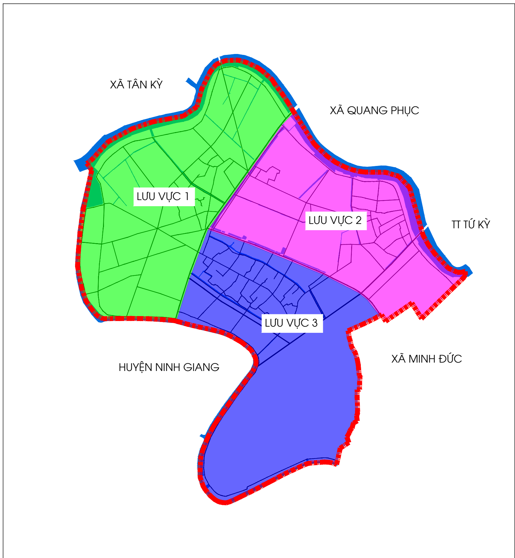
SƠ ĐỒ PHÂN LƯU VỰC THOÁT NƯỚC
